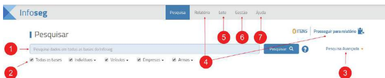
Figura 10: Tela Inicial
