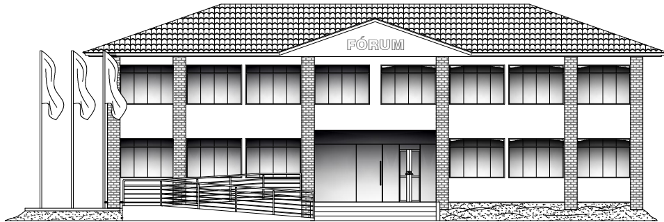
FACHADA FRONTAL
