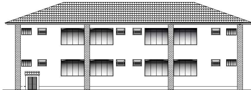
FACHADA POSTERIOR
