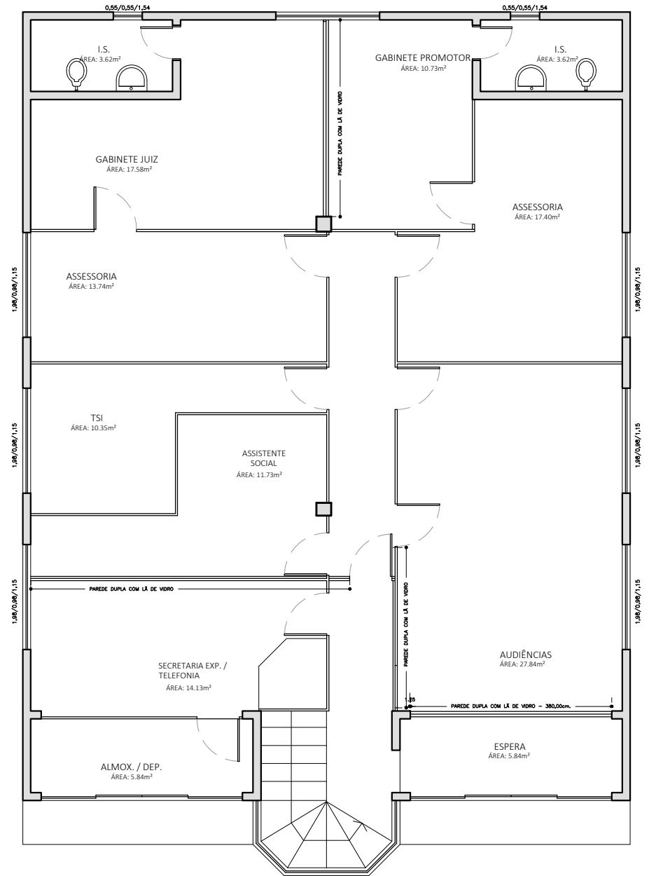
PAVIMENTO SUPERIOR
