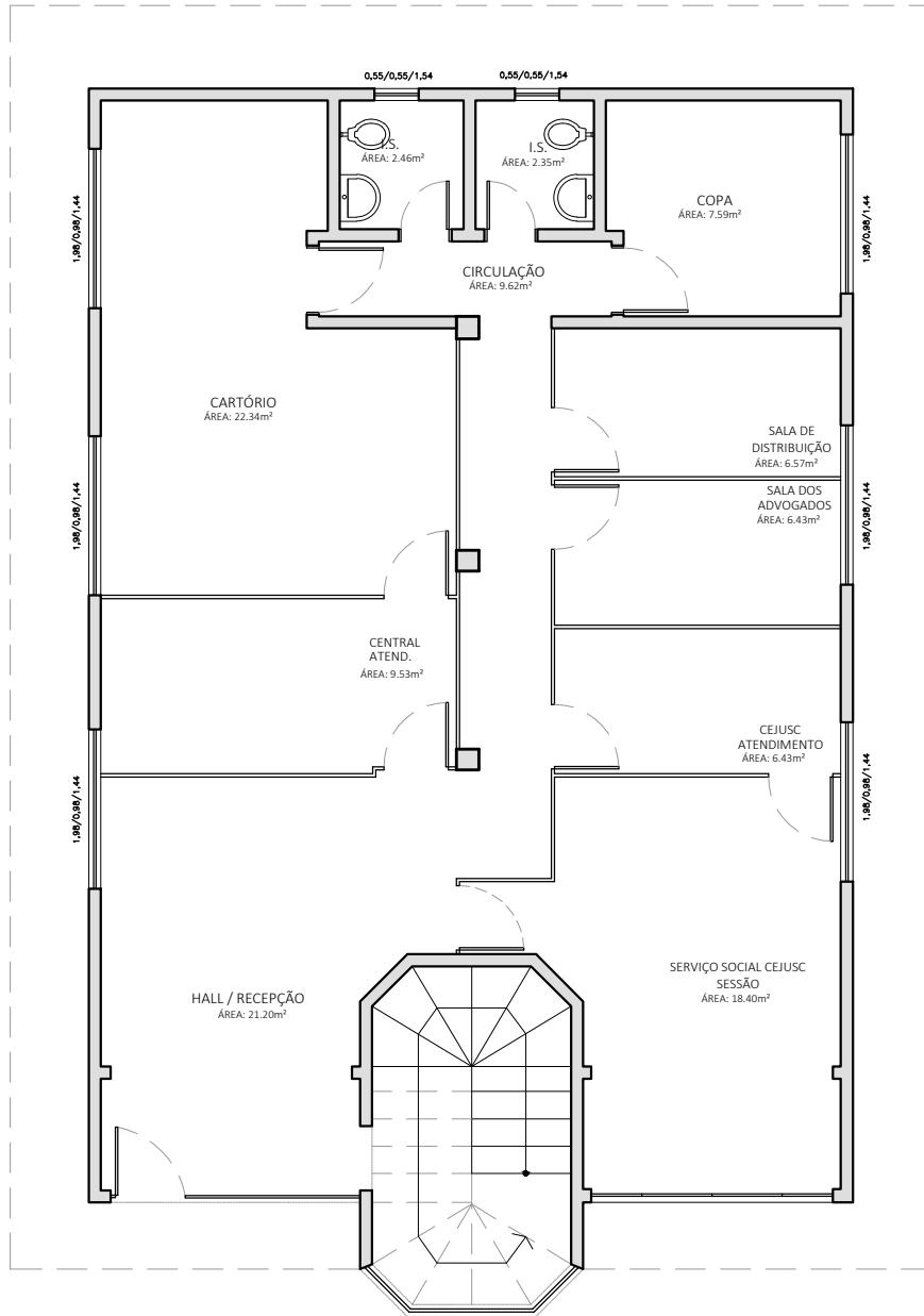
PAVIMENTO TÉRREO
